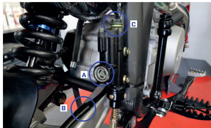
A : Réservoir du liquide de frein / B : Durite de frein / C : Vis du bouchon de réservoir
