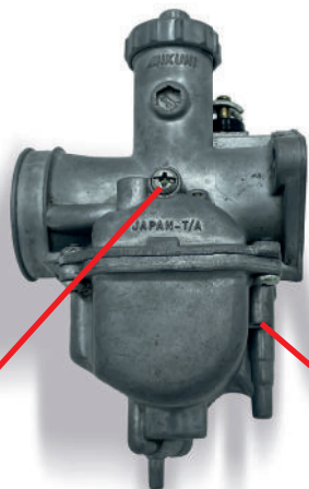
Vis de ralenti
