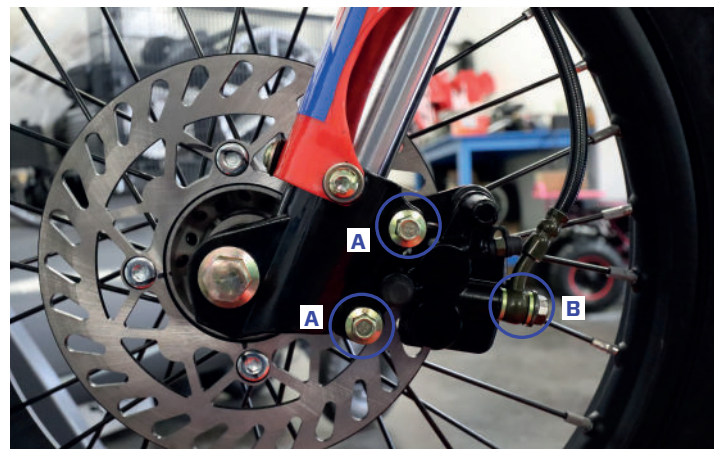
(A) Écrous de fixation de l'étrier du frein (B) Étrier
